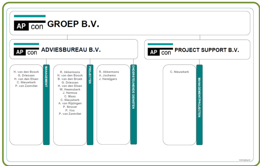
Figuur 1 – Organisatiegrenzen
